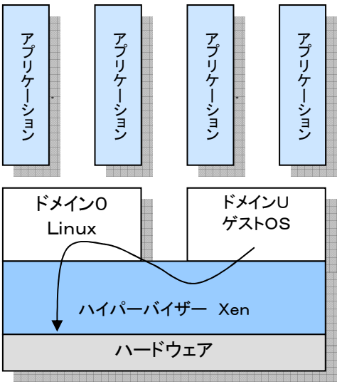
Xen
